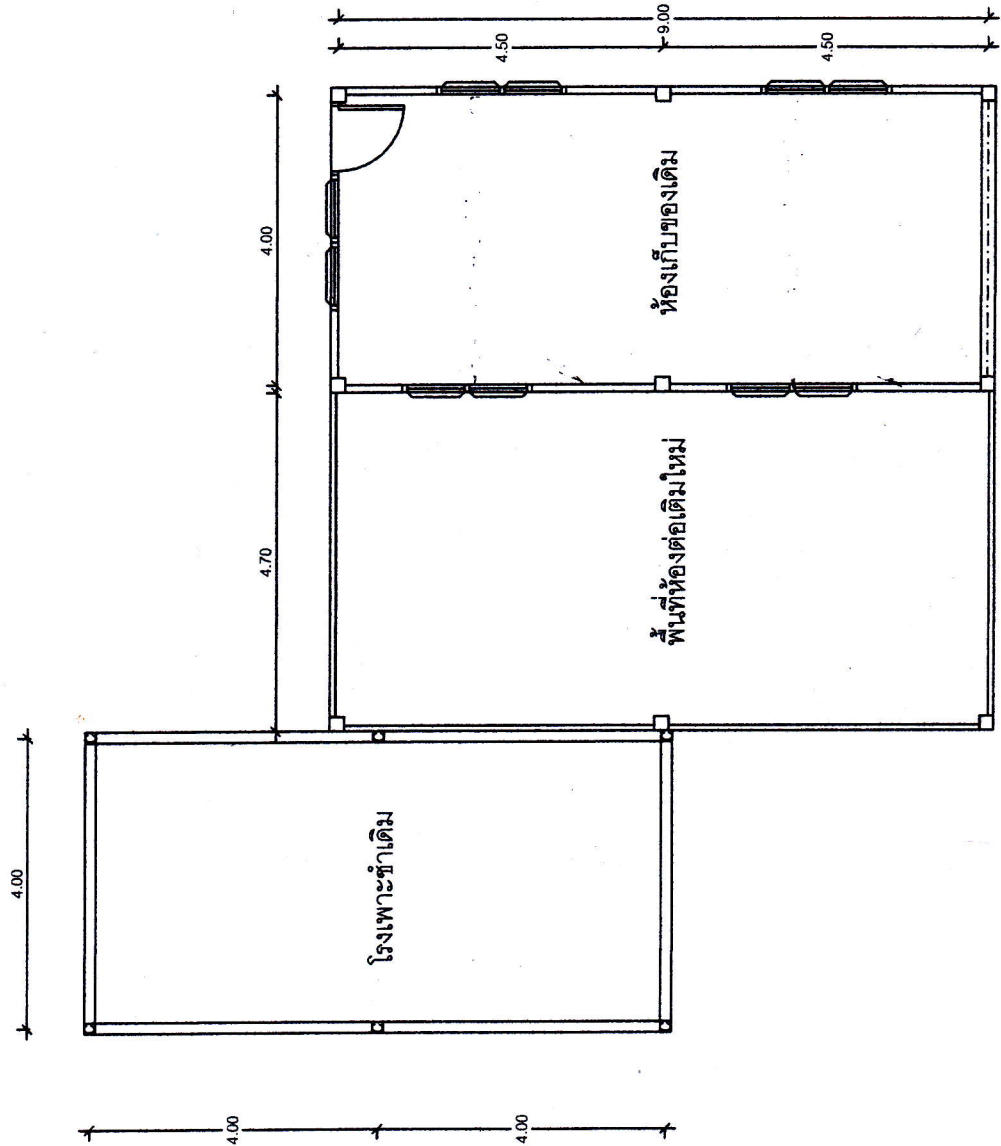
แปลนส่วนขยายและห้องเก็บของปรับปรุงใหม่ 1:75
